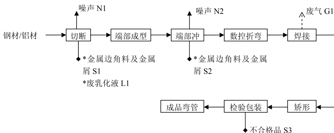
图 5-1 汽车内饰弯管生产工艺流程图
