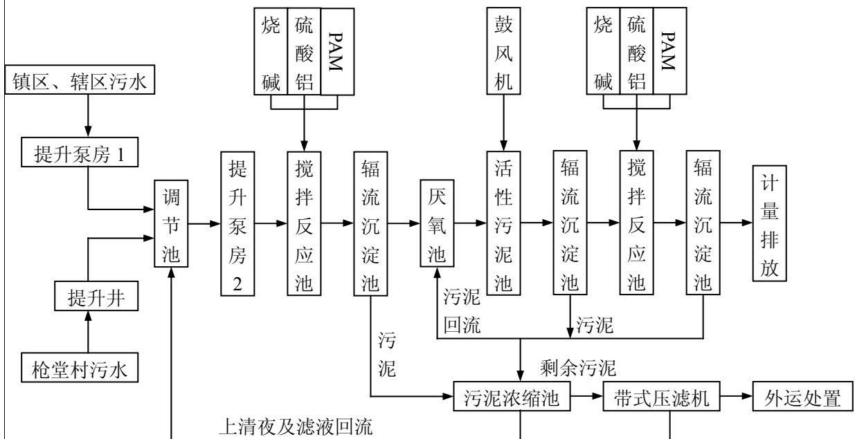
图 7-1 污水厂污水处理工艺流程图
